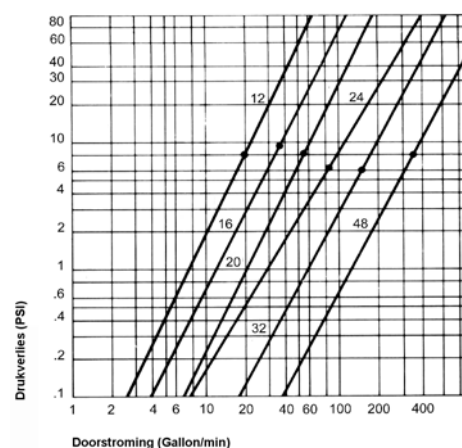
Drukverlies - Doorstroming
